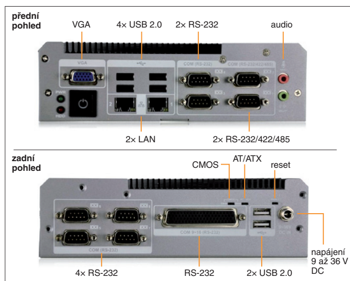
Obr. 2. Rozhraní vestavného počítače TANK-600
