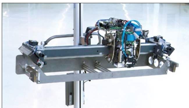
Obr. 2. Výměnný portál linky Siplace SX
