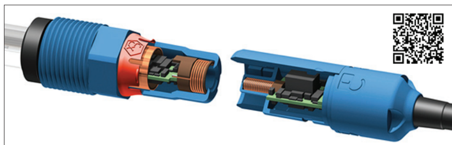
Obr. 1. Senzory Memosens digitalizují měřenou hodnotu a přenášejí ji indukční vazbou v bajonetové spojce (video: https://youtu.be/f17DyeCMas4 )
