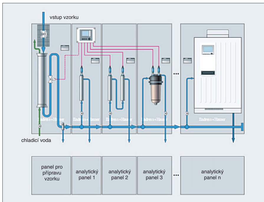
Obr. 3. Schéma modulárního panelu SWAS
