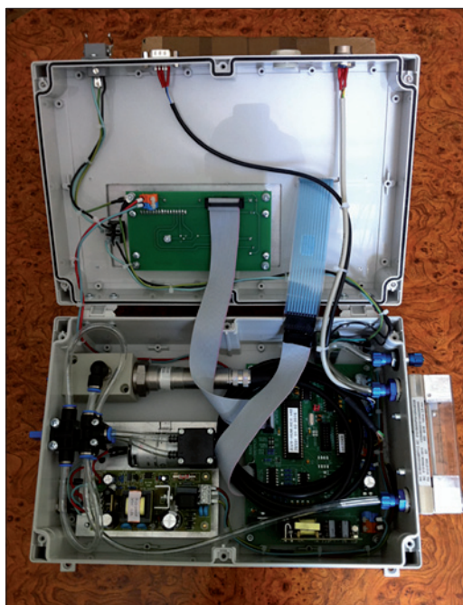
Obr. 4. Vnitřní uspořádání analyzátoru vlhkosti System 1211FP (na víku: síťová vidlice napájení 230 V 50 Hz, datový konektor RS-232C, konektor analogových výstupů 3 × 4 až 20mA; spodní díl skříňky: průtočná komůrka s měřicí sondou, membránové čerpadlo s napájecím zdrojem, mikroprocesorová elektronika analyzátoru, propojení pneumatického obvodu s ventilem obtoku čerpadla a plovákový průtokoměr)
